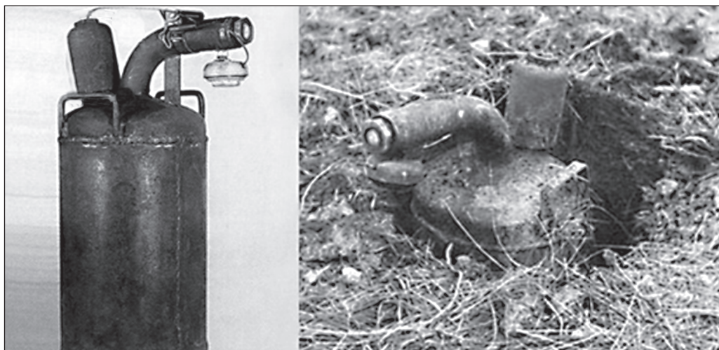
Огнемёт ФОГ-1. Фото из открытых источников*
