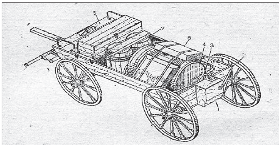
Дегазационная повозка КДП-250.
