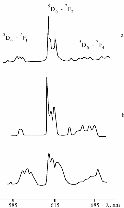
Рис.1. Спектры люминесценции (77К) комплексов европия: а- [Eu(Тол)_3 \cdot dipu]_2 , б- Eu(Кор)_3 \cdot 2phen \cdot H_2O , с- Eu(ТФА)_3 \cdot ДФА \cdot 2 H_2O
