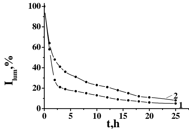
Рис.6. Зависимость интенсивности люминесценции композиций [\text{Eu}(\text{TFA})_3 \cdot \text{dipy} \cdot 3\text{H}_2\text{O}] \cdot \text{dipy} + \text{АНТ} в ПЭВД от времени облучения УФ светом: 1 - мольное соотношение 1:0,5; 2 - мольное соотношение 1:3
