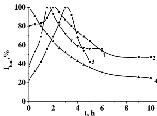
Рис.2. Зависимость интенсивности люминесценции европия от времени облучения УФ светом: а - 1-Eu(Кор) 3 ·2dipy·H 2 O, 2-[Eu(ТФА) 3 ·dipy·3H 2 O]dipy, 3-Eu(NO 3 ) 3 ·phen, 4-[Eu(Тол) 3 ·dipy] 2 ; б -1-Eu(Кор) 3 ·2phen·H 2 O, 2-[Eu(Тол) 3 ·phen] 2 , 3-Eu(ТФА) 3 ·2phen·H 2 O, 4- Eu(NO 3 ) 3 ·phen
