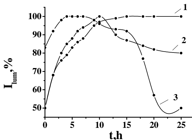
Рис.5. Зависимость интенсивности люминесценции композиций \text{Eu}(\text{ТФА})_3 \cdot 2\text{phen} \cdot \text{H}_2\text{O} + \text{АНТ} в ПЭВД от времени облучения УФ светом: 1 - мольное соотношение 1:05; 2 - мольное соотношение 1:3; 3 - мольное соотношение 1:6
